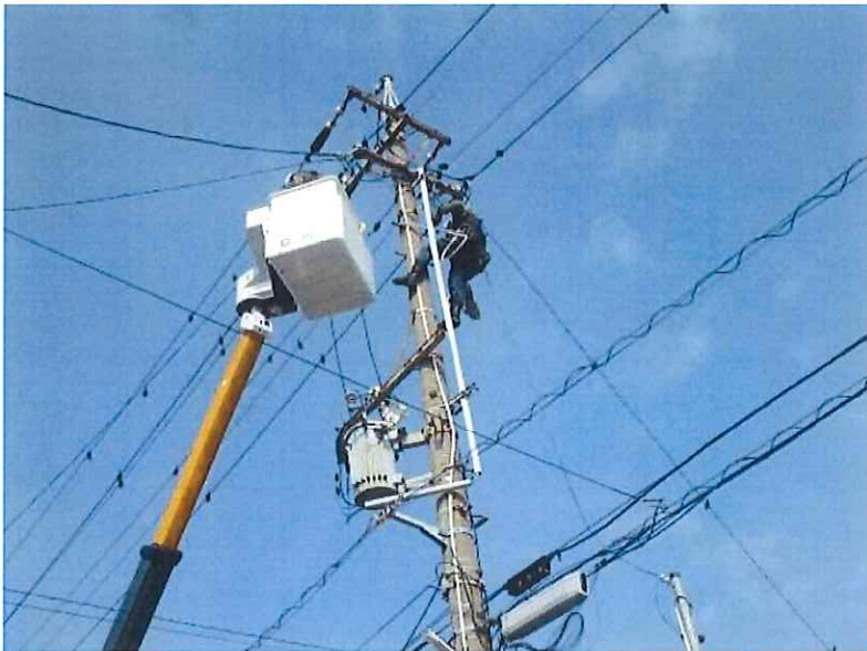
引込柱昇柱 作業状況
